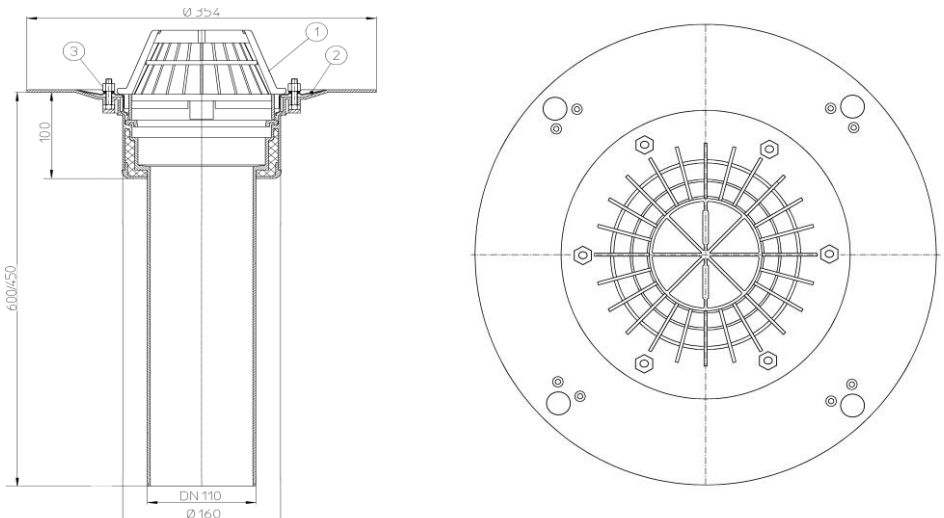
Рис. 1. Чертеж воронки
